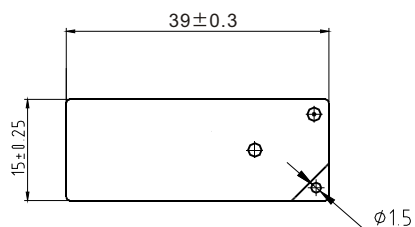
外形尺寸图
