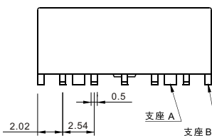
外形尺寸图
