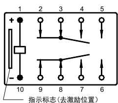
接线图(底视图)
