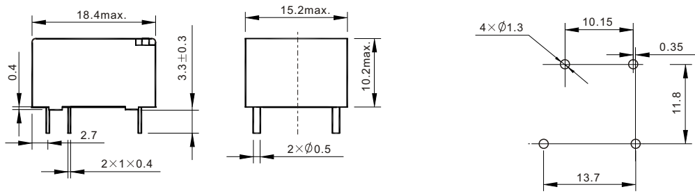
外形尺寸图
