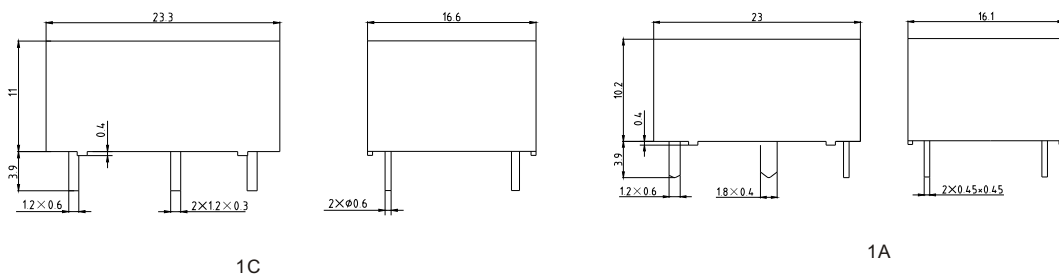
外形尺寸图
