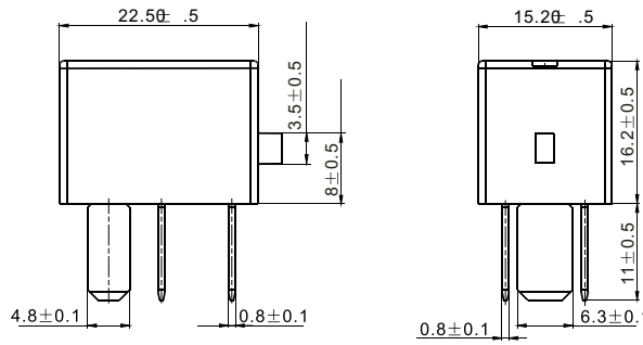
外形尺寸图
