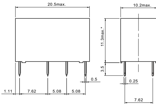
外形尺寸图
