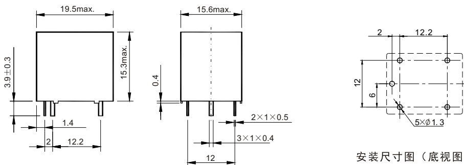
外形尺寸图
