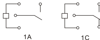
1A 1C 接线图(底视图)
