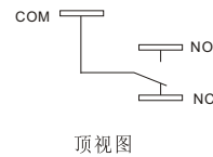
顶视图
